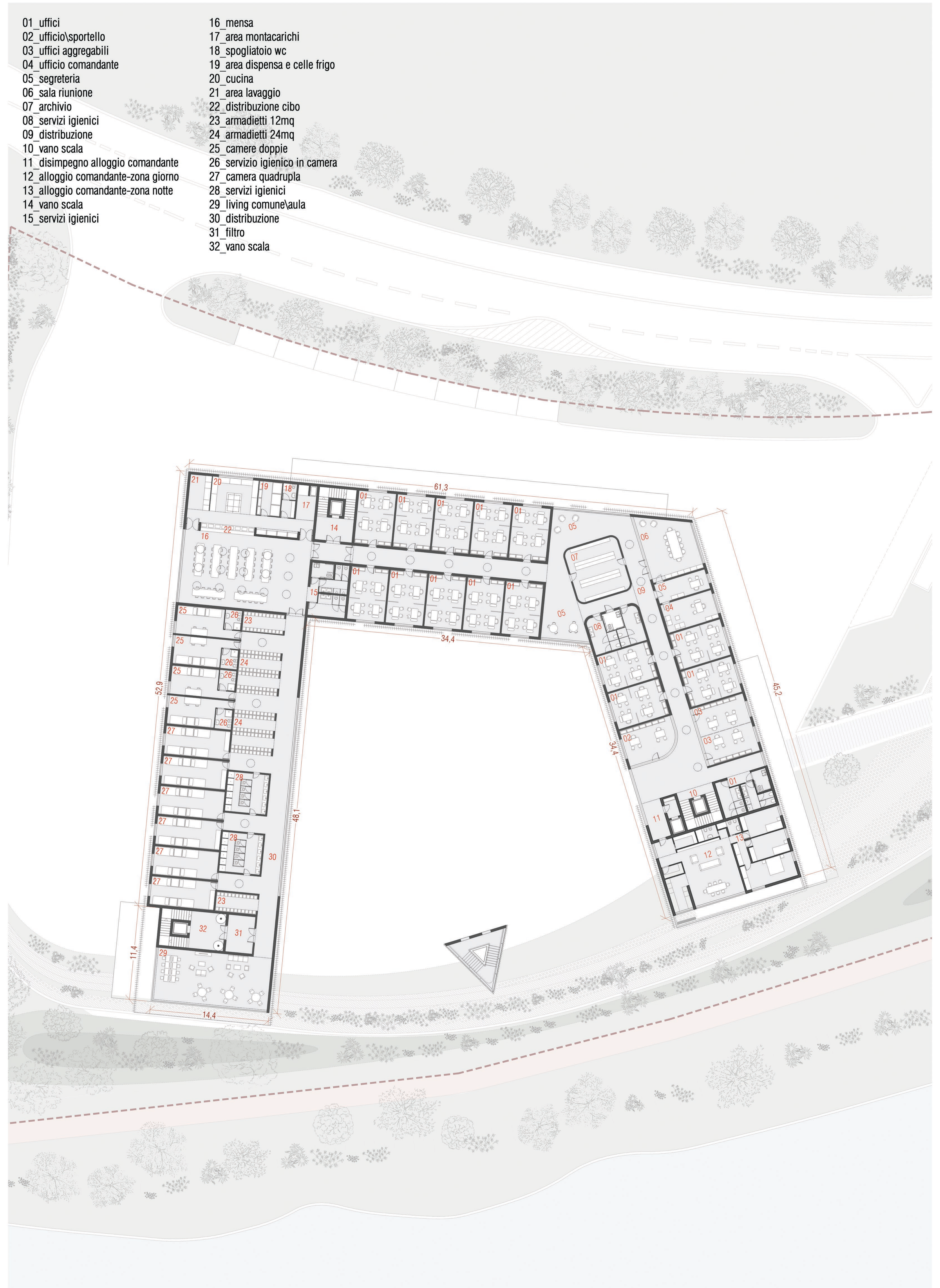
Planimetria primo piano scala 1:200
