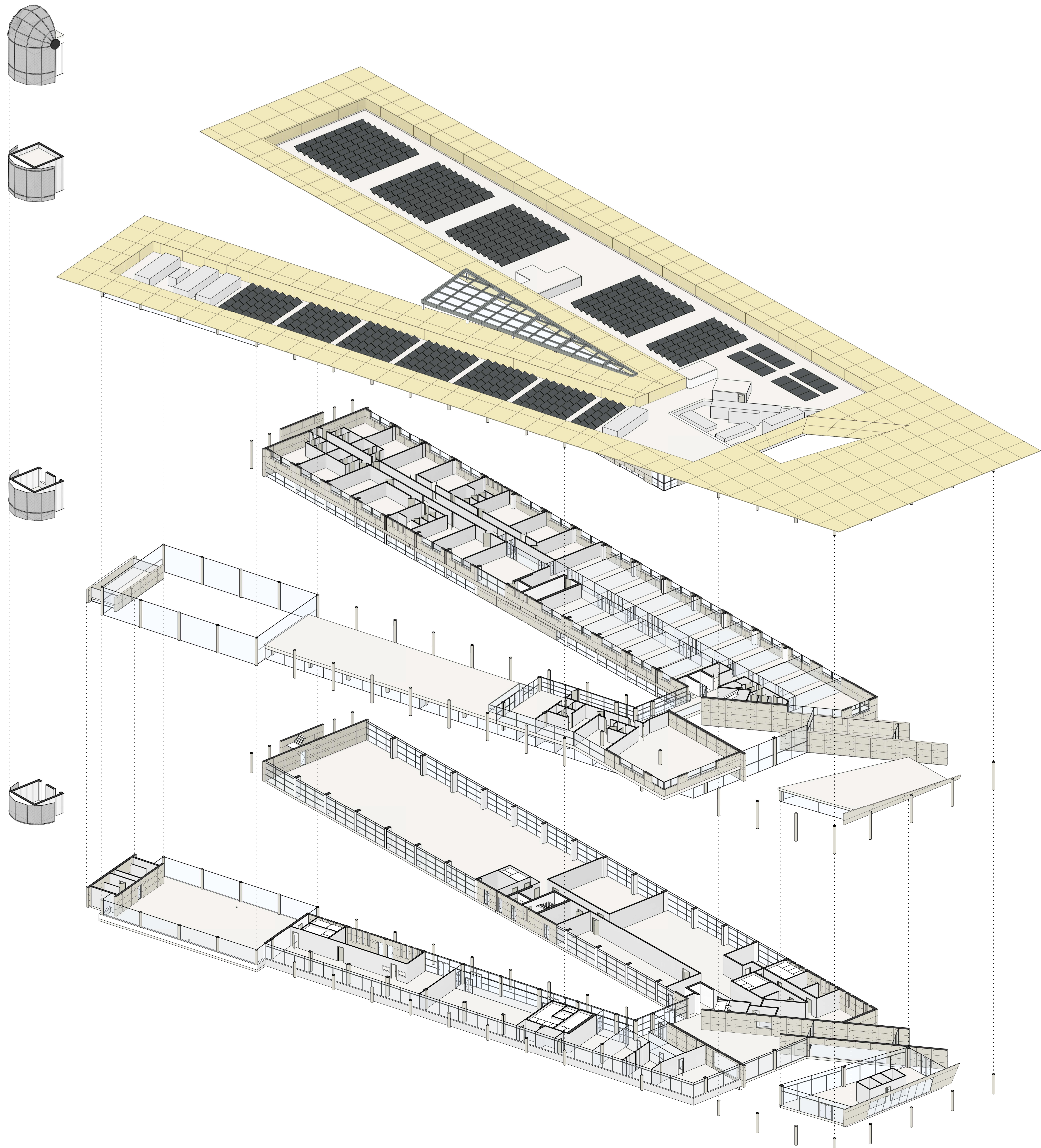
ESPLOSO ASSONOMETRICO Scala 1:200
